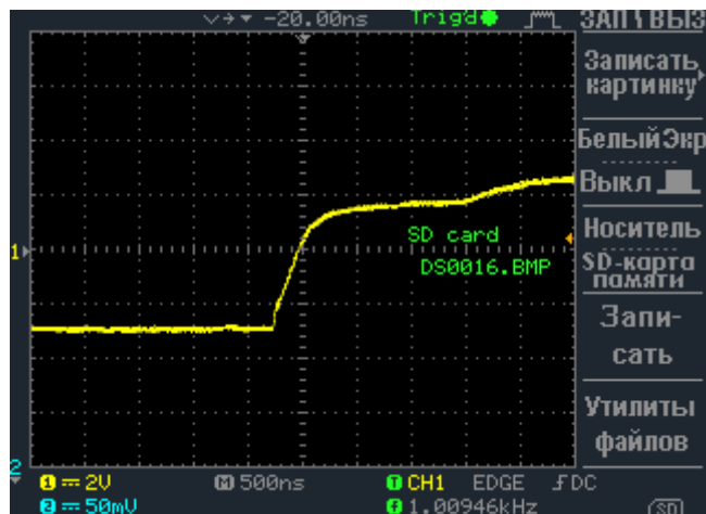
Рисунок 6.3. Линия, согласованная 1 кОм. Видео: enip2.ru/files/rs485_03.zip
