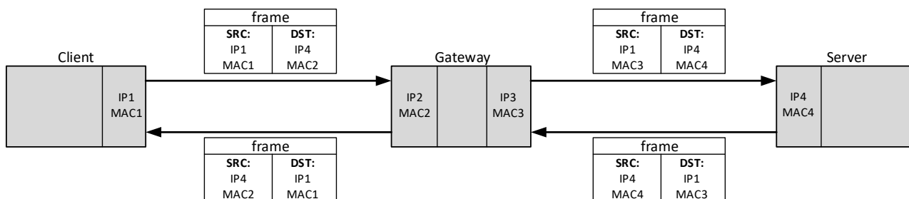
Рисунок 6.5. Пример прохождения кадров при запросе из другой подсети
