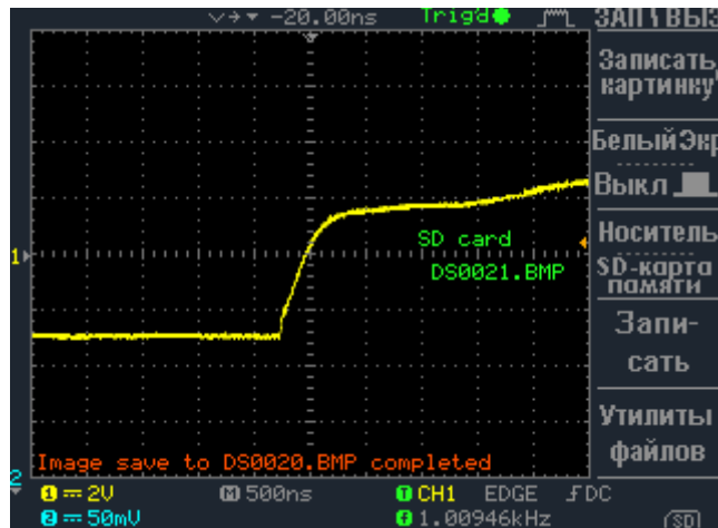
Рисунок 6.4. Линия, согласованная 120 Ом. Видео: enip2.ru/files/rs485_04.zip
