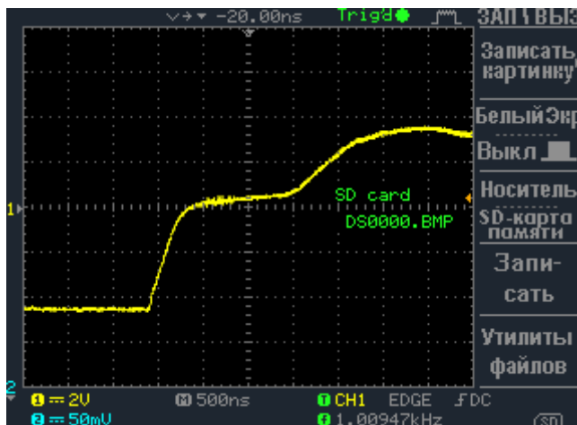
Рисунок 6.1. Несогласованная линия. Видео: enip2.ru/files/rs485_01.zip
