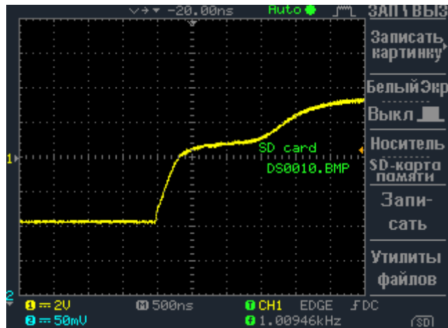
Рисунок 6.2. Линия с «оттяжками» 1 кОм. Видео: enip2.ru/files/rs485_02.zip
