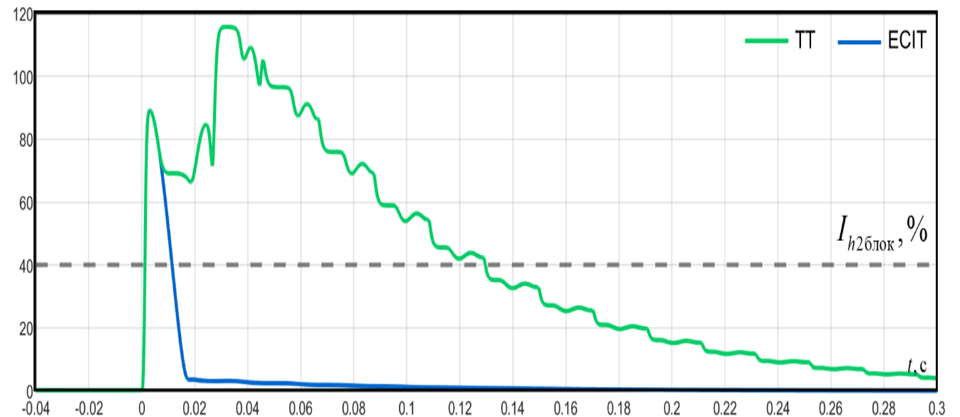
Рис.7 – Вторая гармоника тока при БНТ
